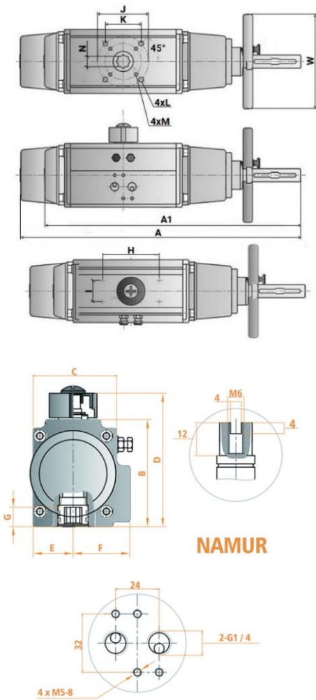
Габаритный чертеж пневмопривода
