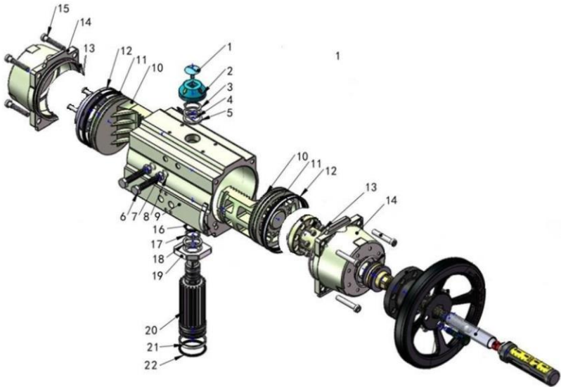
Спецификация. Пневмопривод.
